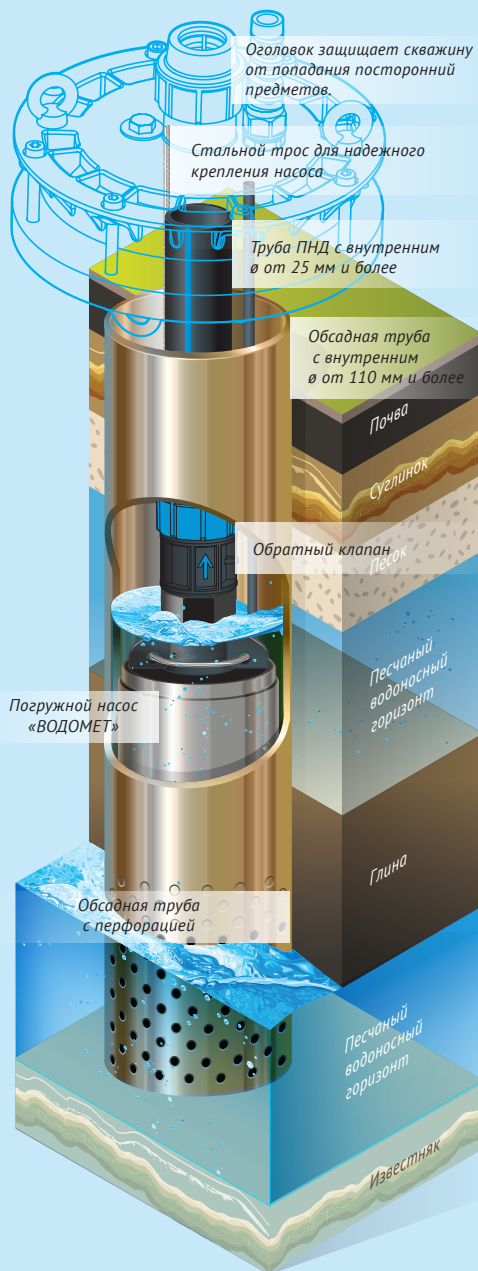
Рисунок 3. Пример установки насоса.
